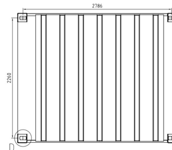
Bovenaanzicht
