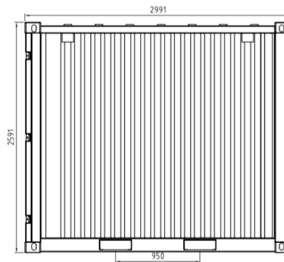
Zijaanzicht
