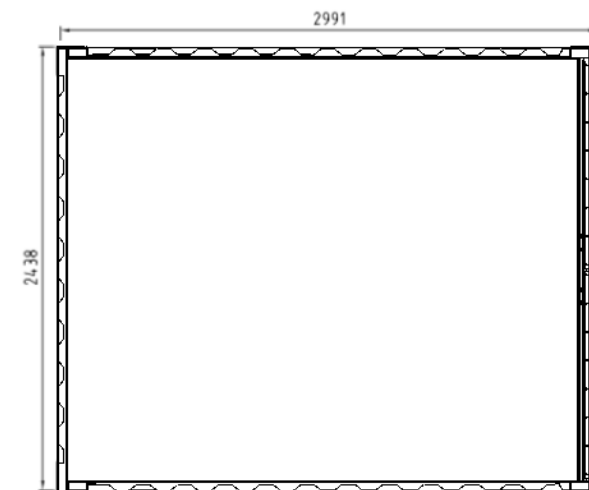
Bovenaanzicht
